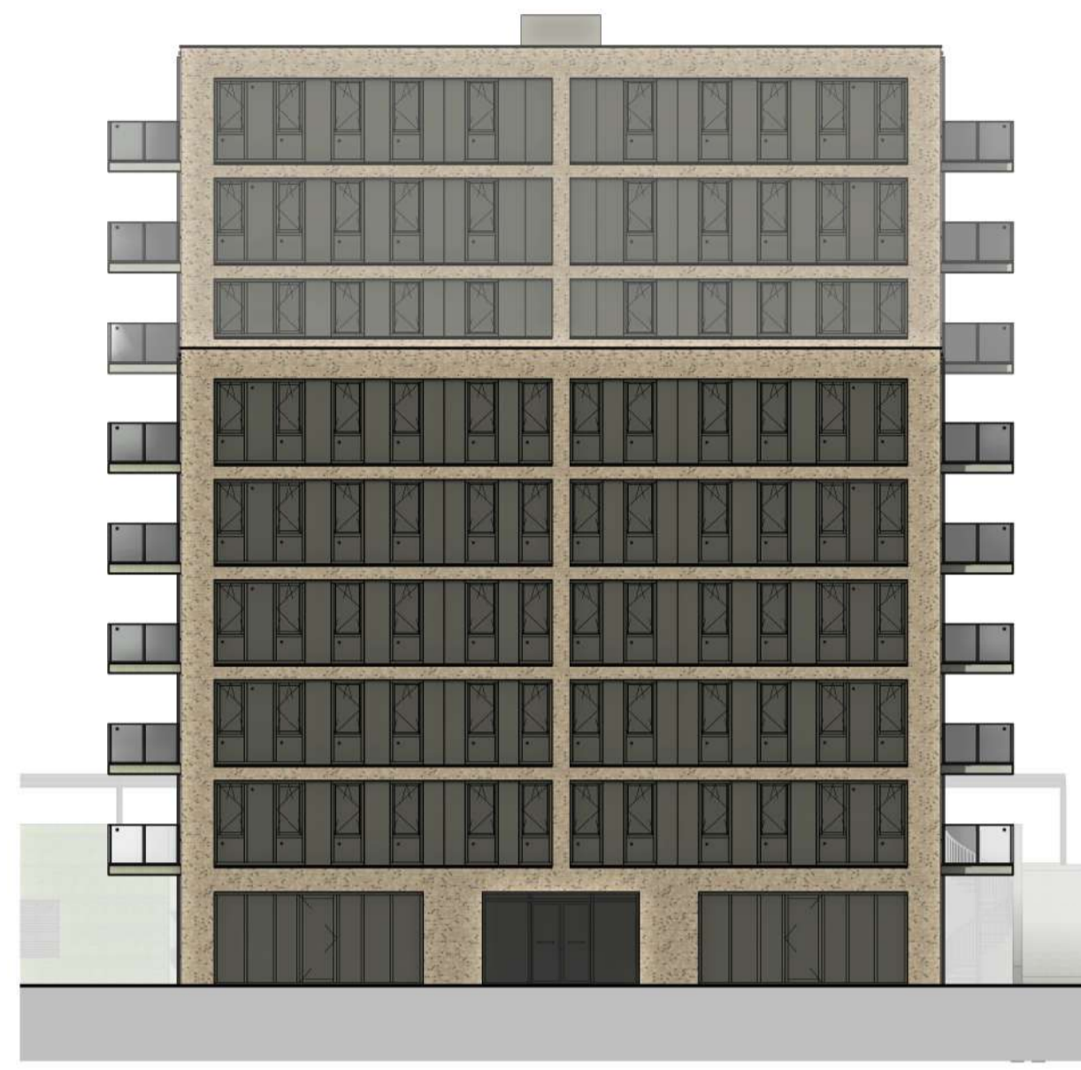
Noordgevel blok B 1 : 200
